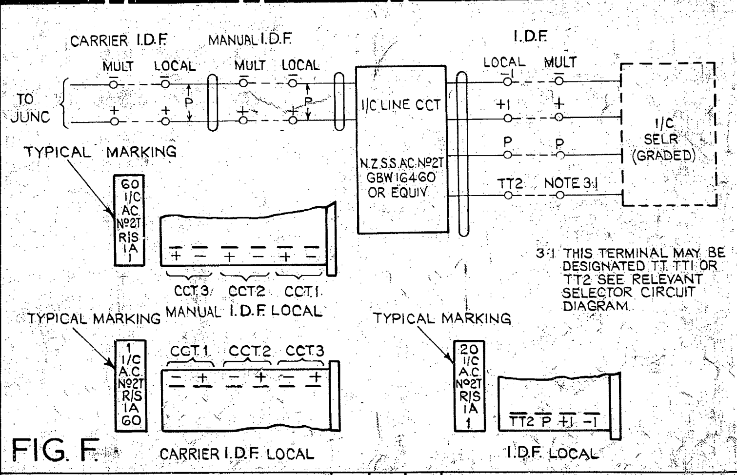
FIG. E. CARRIER I.D.F. LOCAL I.D.F. LOCAL
