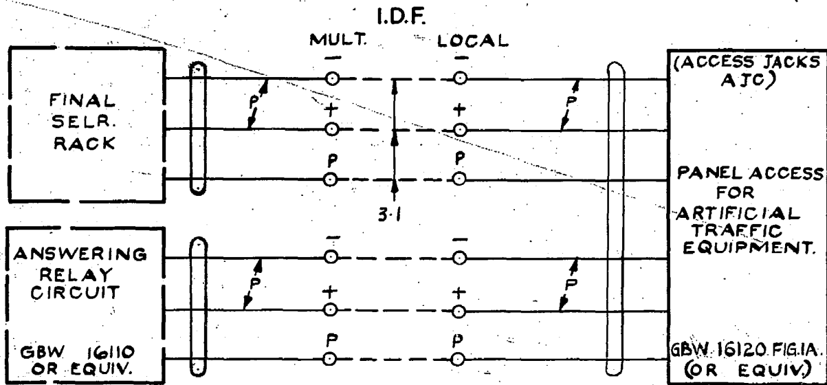
FIG. E. TEST N° CIRCUIT N° 1.
