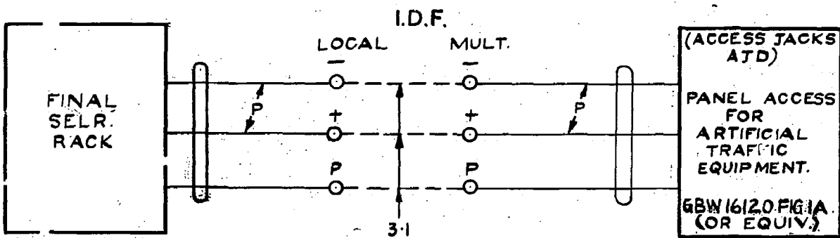
FIG. F. TEST N° CCT N° 1
