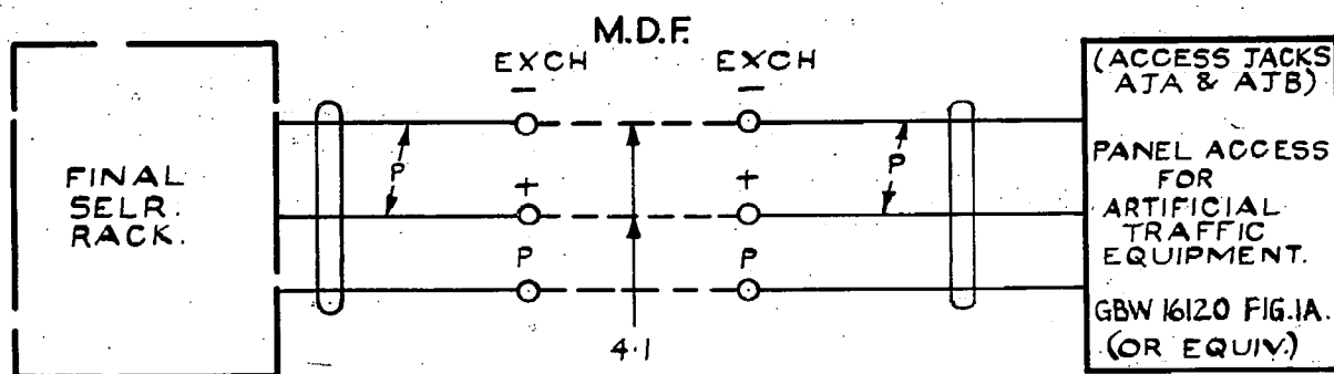
FIG. G. LINE CIRCUIT N o 1.
