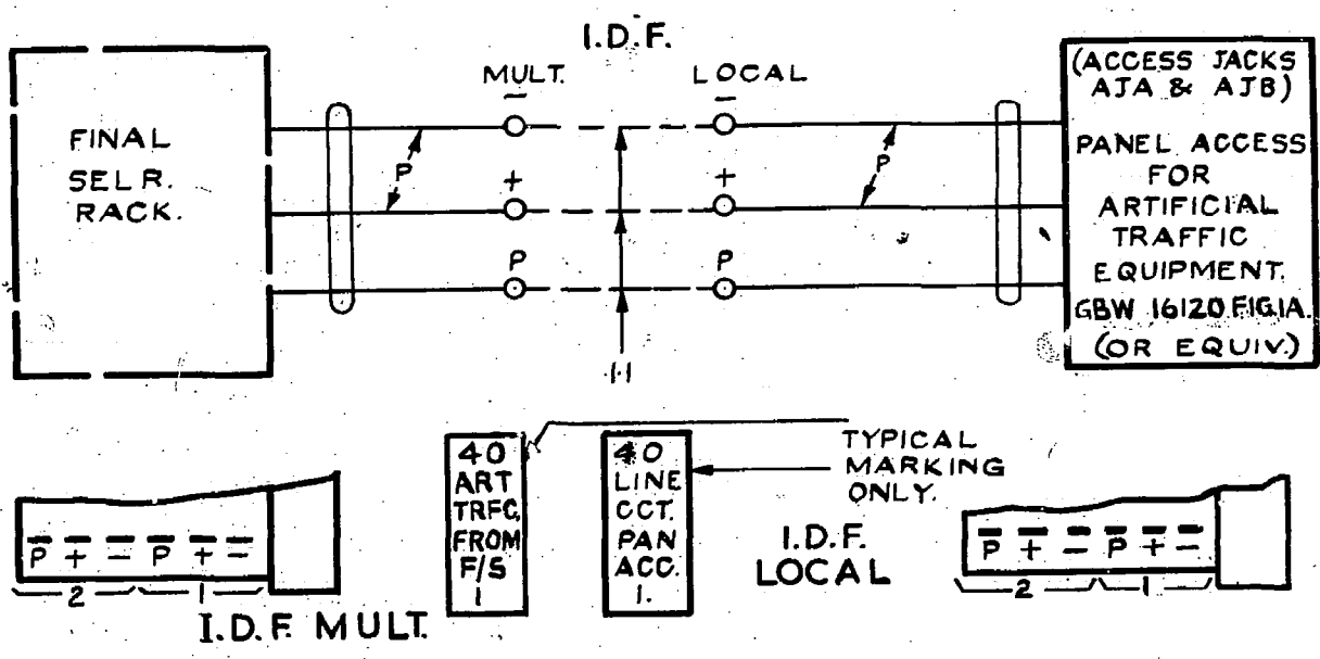
FIG. B. LINE CIRCUIT N°1
