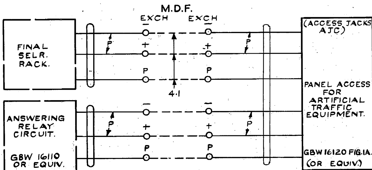
FIG. H. TEST N o CIRCUIT N o 1.
