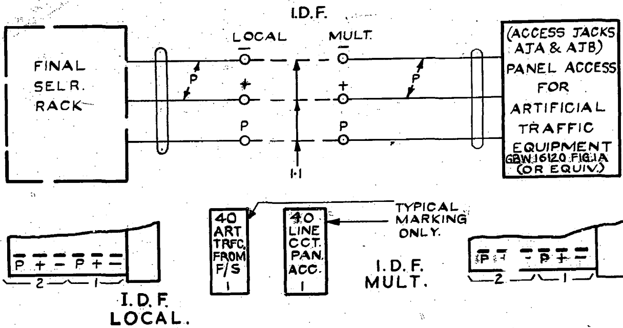
FIG. A. LINE CIRCUIT N°1
