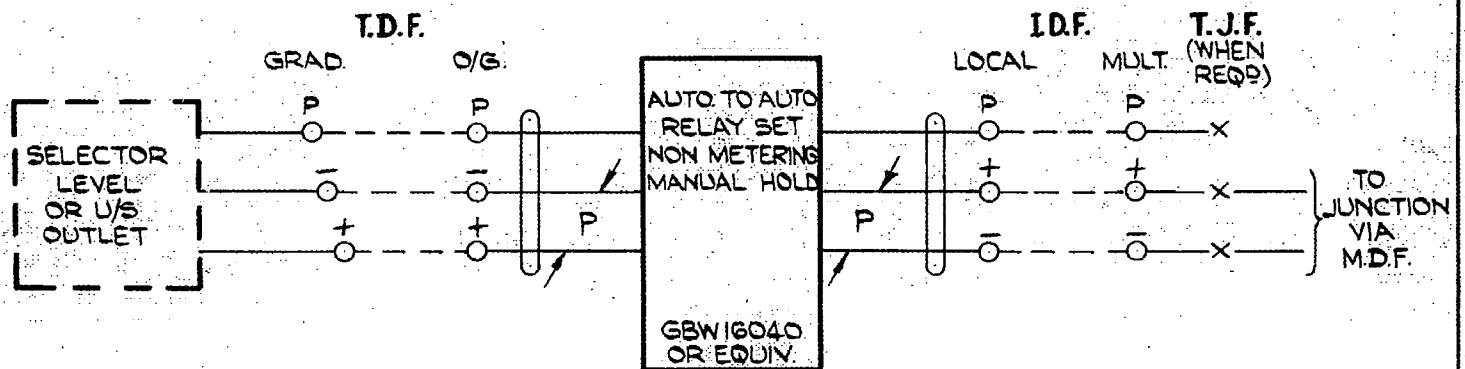
FIG. B INCOMING VIA T.D.F.
