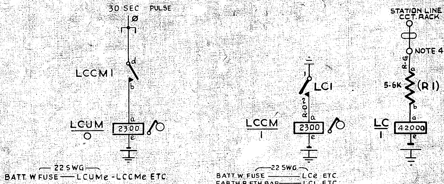
FIG.2. OVERFLOW METER (OM)
