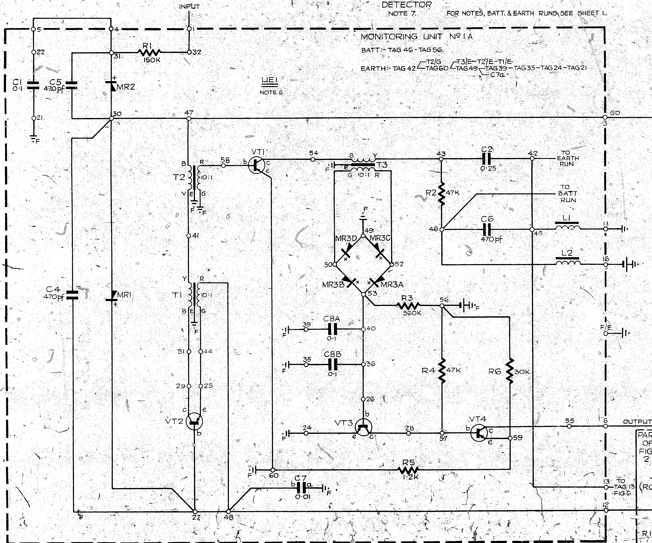
FIG. 5. DETECTOR
