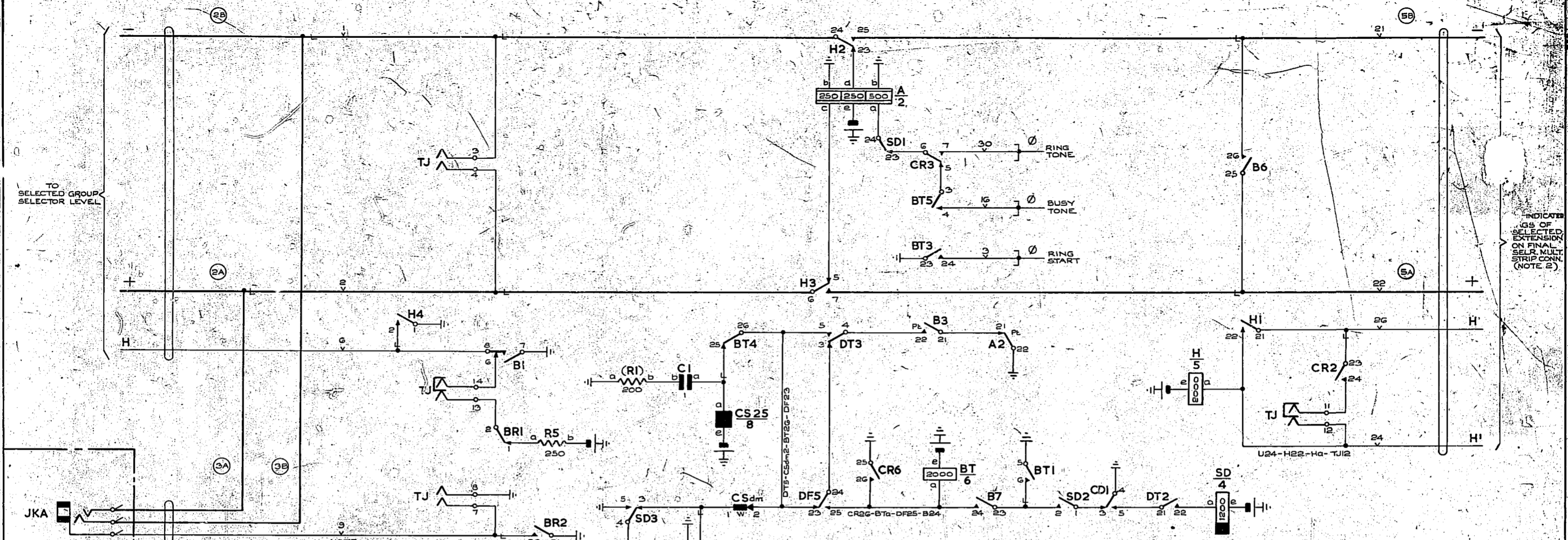
FIG. 1. VISUAL CODE CALL CIRCUIT.
