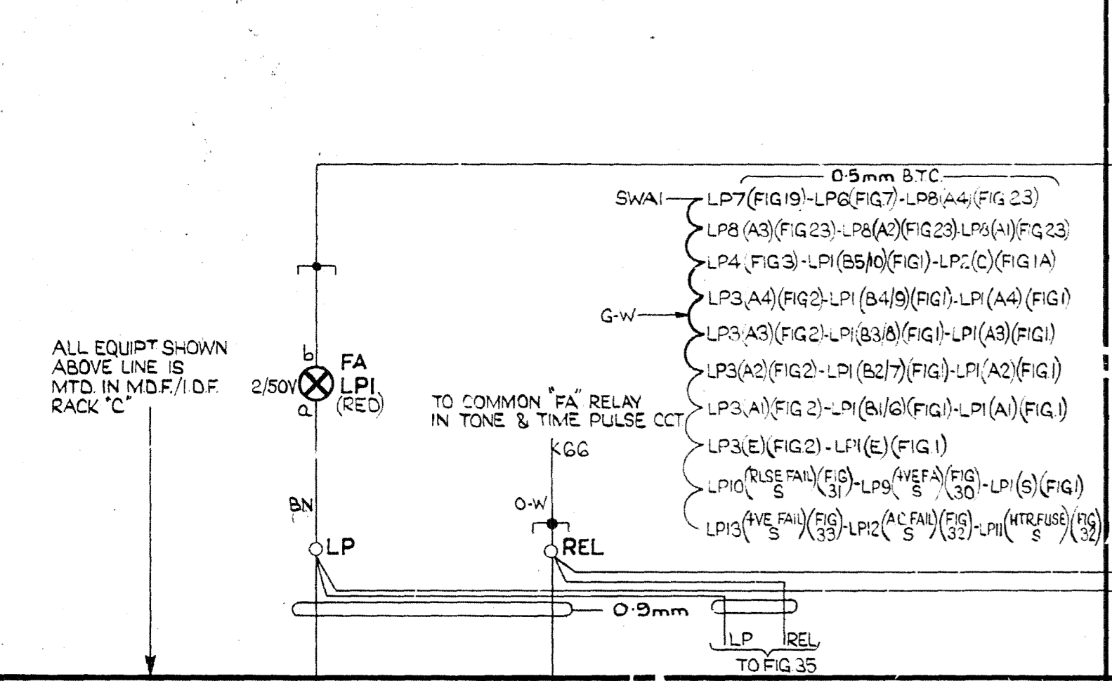
FIG. 1. FUSE ALARM 1 PER UNIT "A" & "S" 1 PER 2 UNITS "B"
