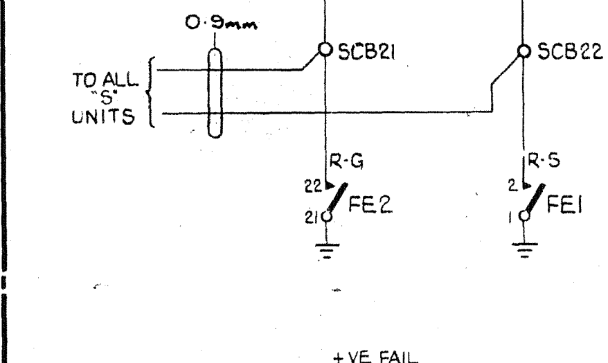
FIG.29A 1 PER 2 UNITS 'B'
