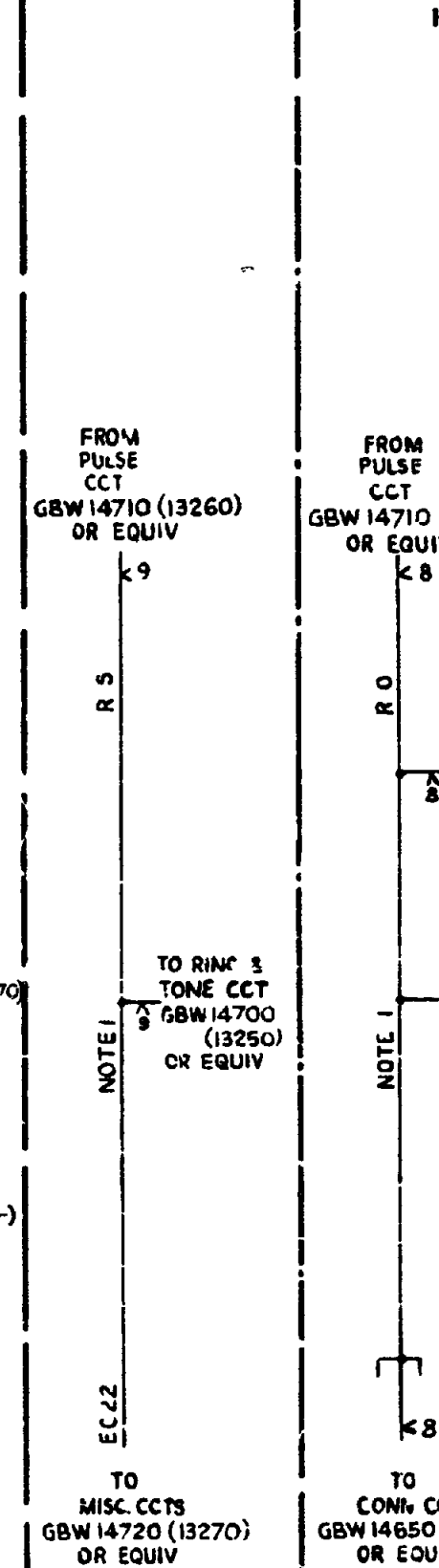
FIG 5 PULSE START 1 PER P A B X
