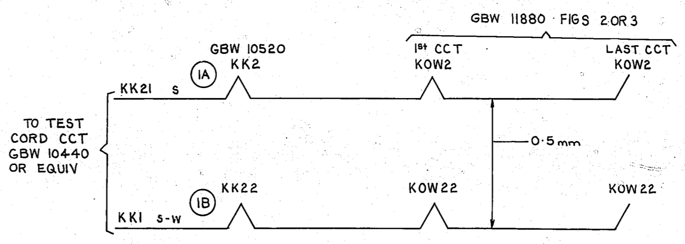
FIG B. TEST CORD CIRCUIT COMMONS
