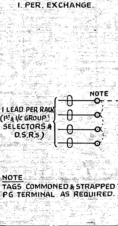
FIG. 1 A.E.R. STRIP CONN.
