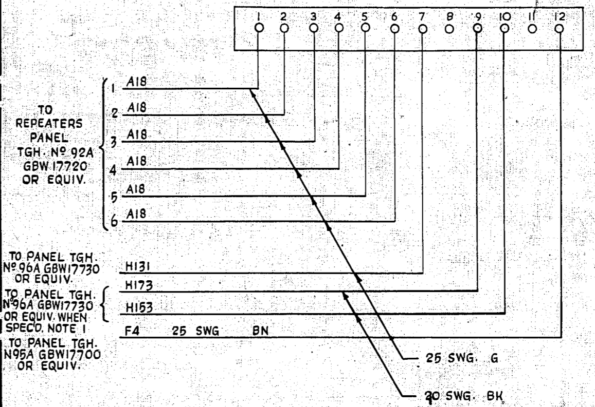
FIG. 3. STRIP CONNEXION E
