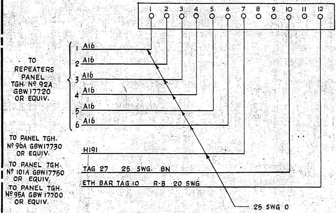
FIG. 2. STRIP CONNEXION D
