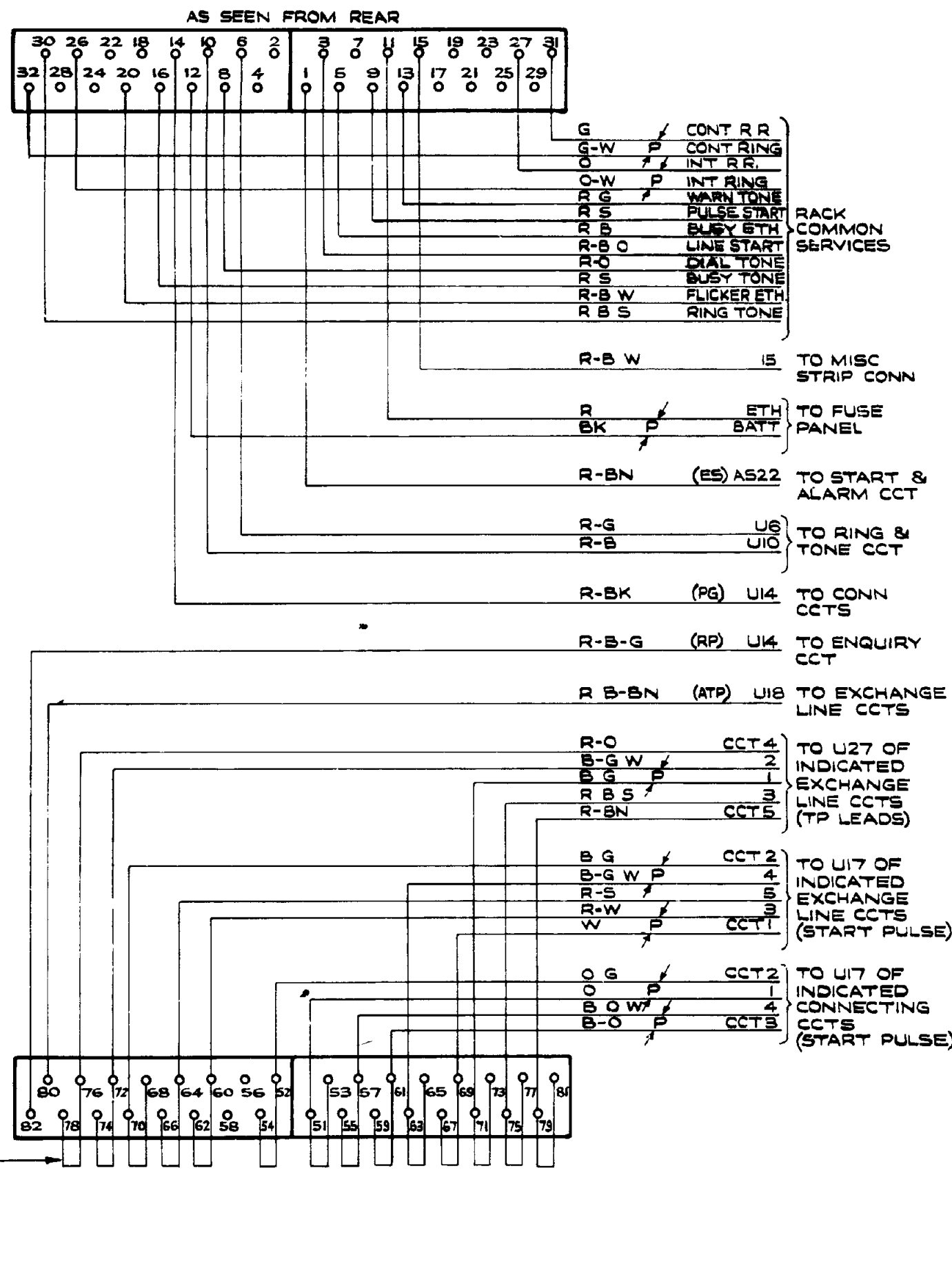
FIG. 1A 20-LINE PABX
